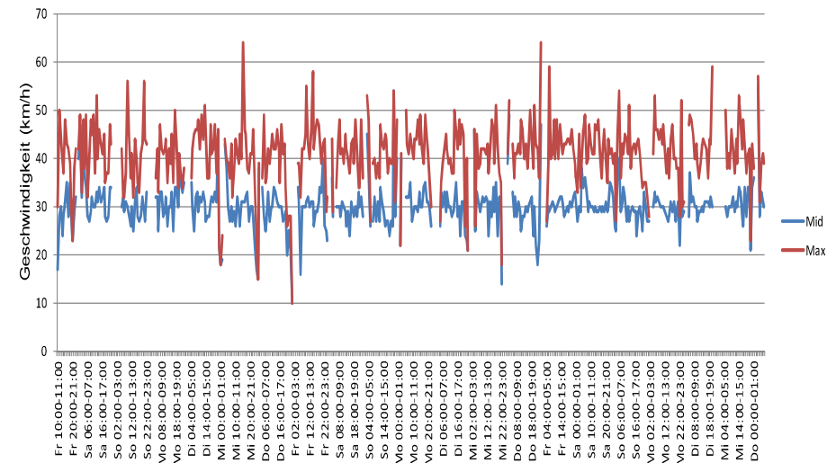
Verlauf Mittlere und Maximale Geschwindigkeit
